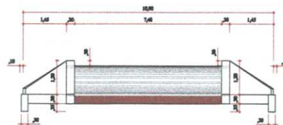
SECÇÃO TRANSVERSAL BUEIRO DN 60 SEM ESCALA
